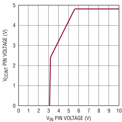
V_{CCINT} vs V_{IN}
