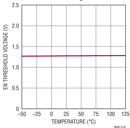
EN Threshold Voltage
