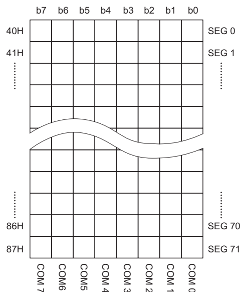
HT56R678 Memory Map – 72×8
