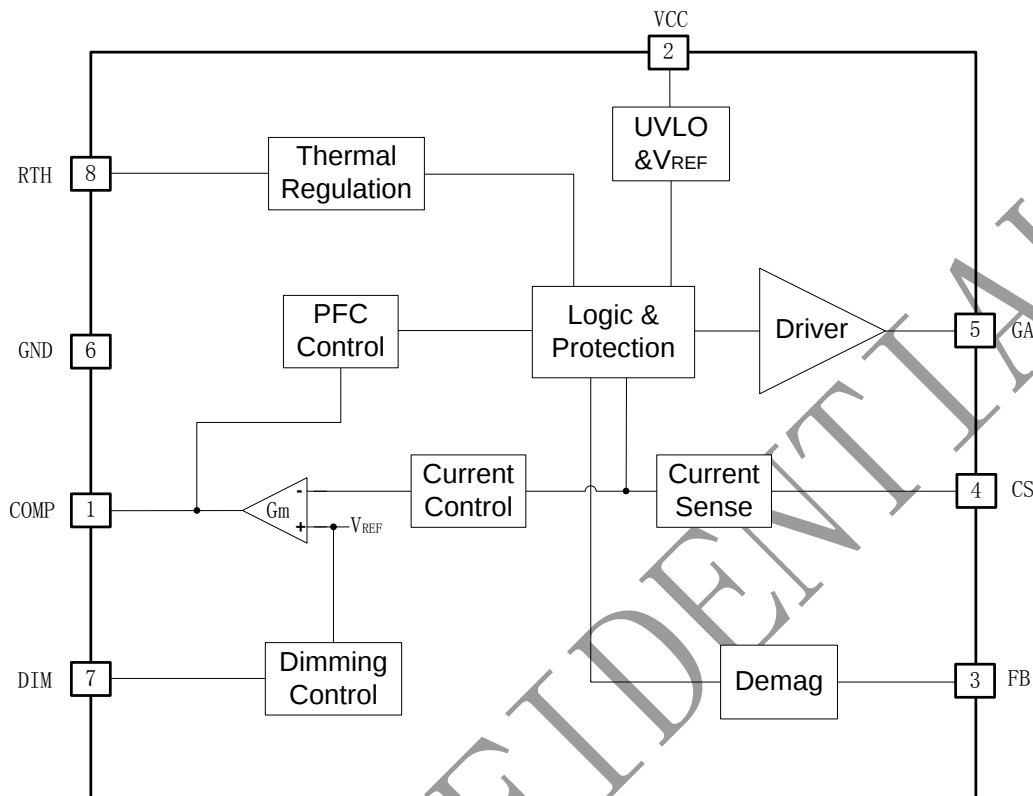
图 3 BP3318 内部框图
