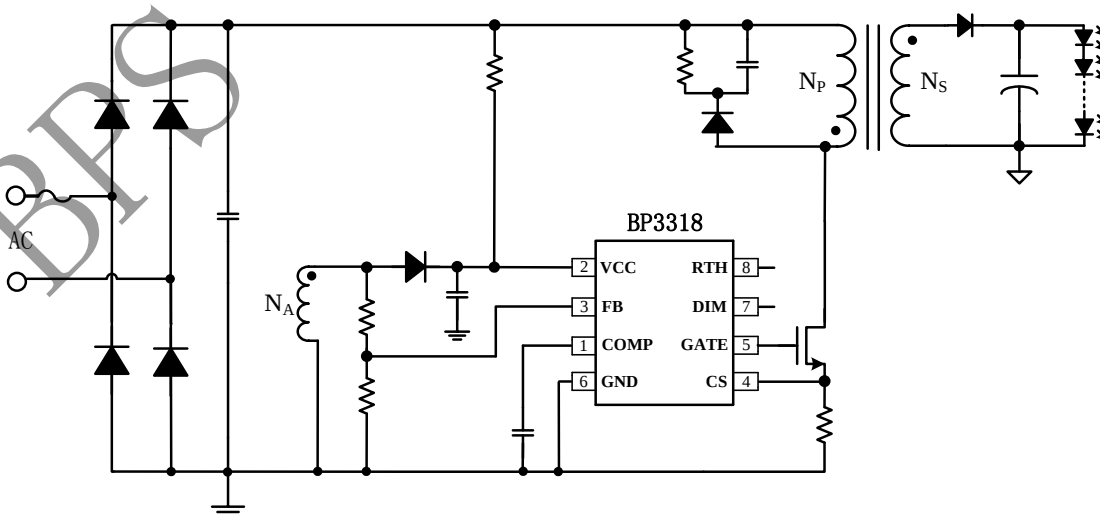
图 1 BP3318 典型应用图
