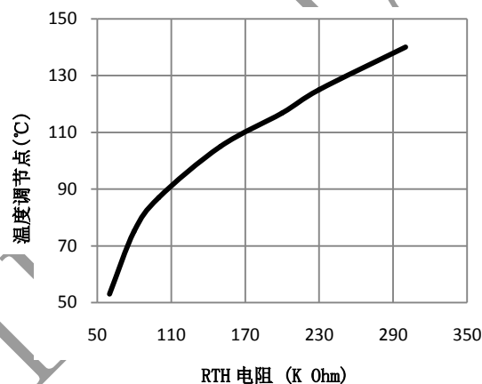
芯片温度调节点与 RTH 电阻的关系
