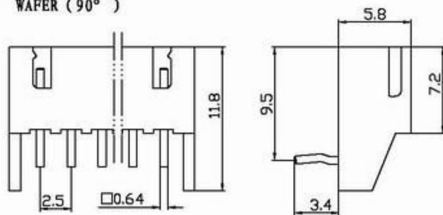
阳连接器 (弯式) WAFER (90°)
