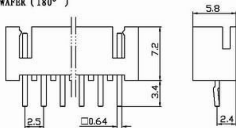
阳连接器 (直式) WAFER (180°)
