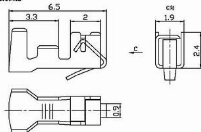
端子 TERMINAL
