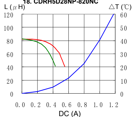
18. CDRH5D28NP-820NC
