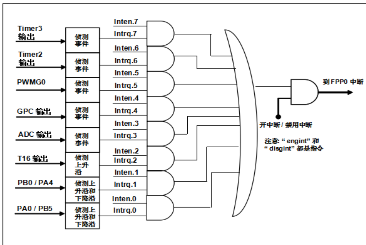
图 16: 中断控制器硬件框图
