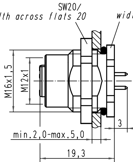
Montageausschnitt/ panel cut out
