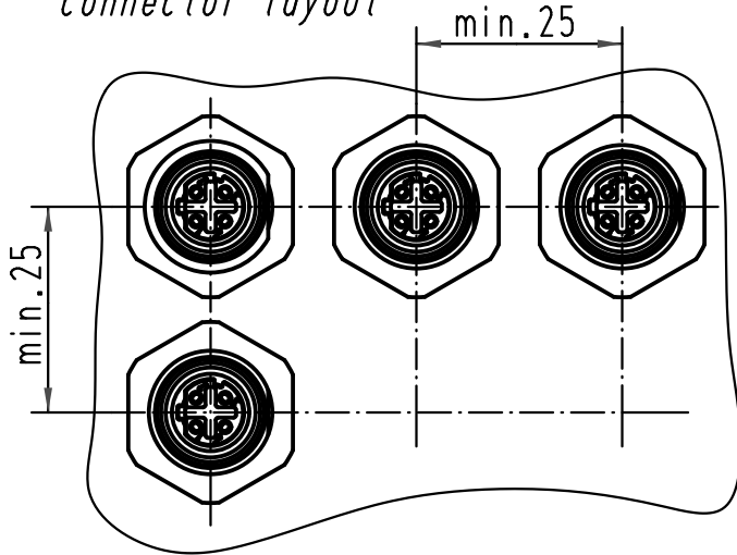
Steckverbinderanordnung/ connector layout
