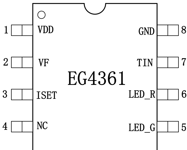
图 4-1. EG4361 管脚定义
