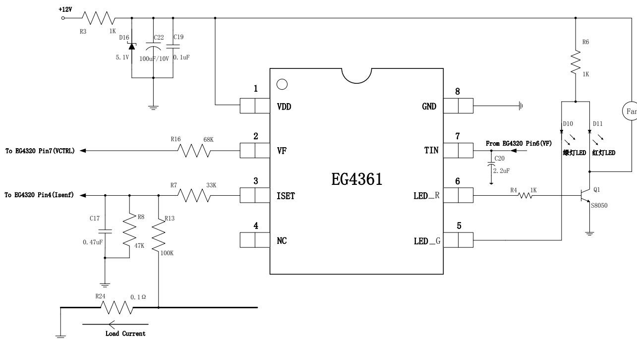
图 6-1a. EG4361 充电器定时控制应用电路图
