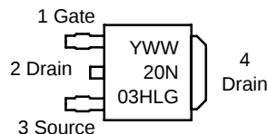
DPAK CASE 369C STYLE 2
